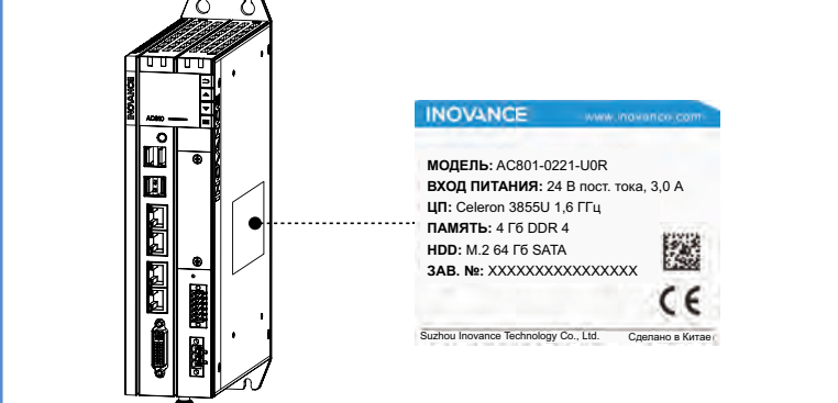
Рисунок 1 Описание номера модели и паспортной таблички
