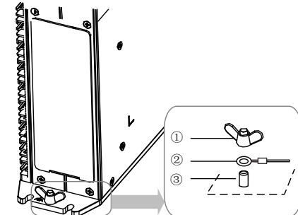
1 – барашковая гайка; 2 – кабель заземления; 3 – винт заземления
