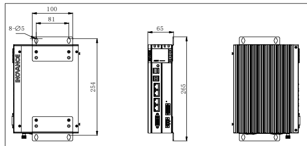
Рисунок 4 Размеры контроллера (боковой кронштейн с проушинами) (в мм)
