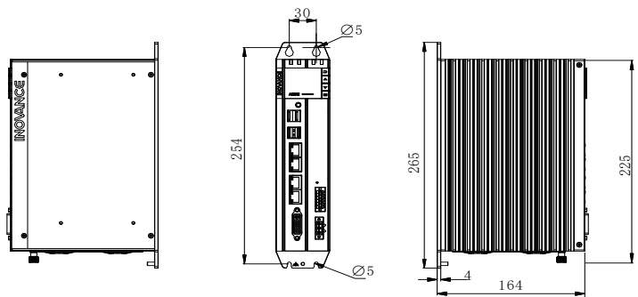
Рисунок 3 Размеры контроллера (задний навесной кронштейн с проушинами) (в мм)
