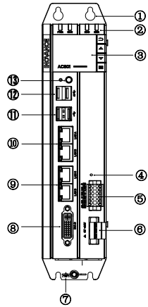
Рисунок 2 Схема интерфейсов контроллера
