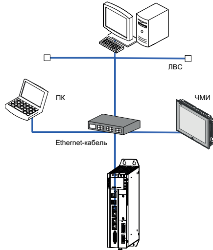
Рисунок 9 Подключение контроллера к другим устройствам через коммутатор
