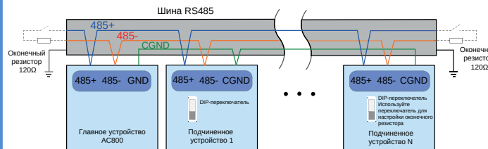
Рисунок 6 Схема подключения к каналу связи RS485
