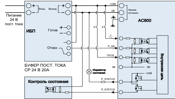
Рисунок 10 Подключение ИБП
