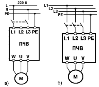
Рисунок 2 - Схема подключения ПЧВ1 и ПЧВ2: а) с однофазным входом 1×220В, б) с трехфазным входом 3×380В
