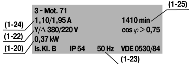
Шильдик двигателя (пример). В скобках указаны номера параметров для ввода в ПЧВ
