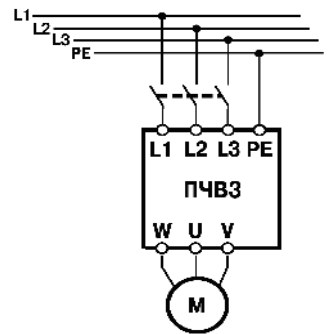
Рисунок 2 - Схема подключения ПЧВ
