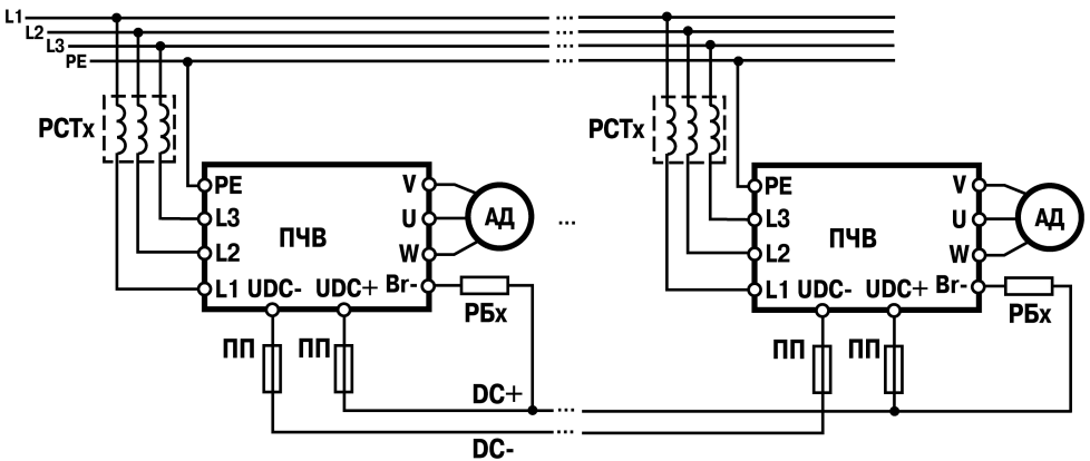
Рисунок 3.5 - Схема разделения нагрузки общей шины постоянного тока
