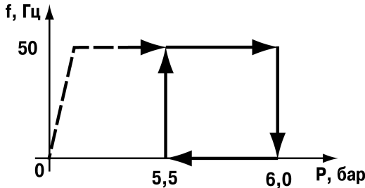
Рисунок 2.5 - Диаграмма релейного режима работы
