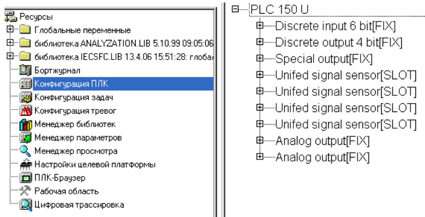
Рисунок 5.1 - Конфигурация ПЛК
