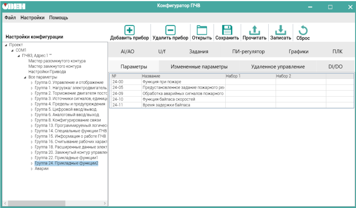
Рисунок 7.2 – Вид рабочего поля меню «Пожарный режим»
